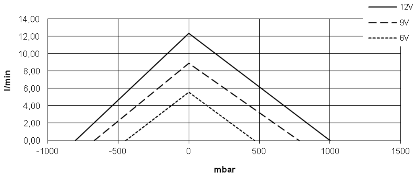
Type/Model: DC12/90KL
