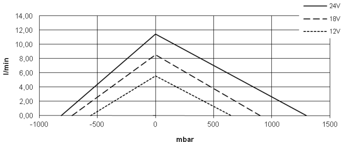
Type/Model: DC24/90L
