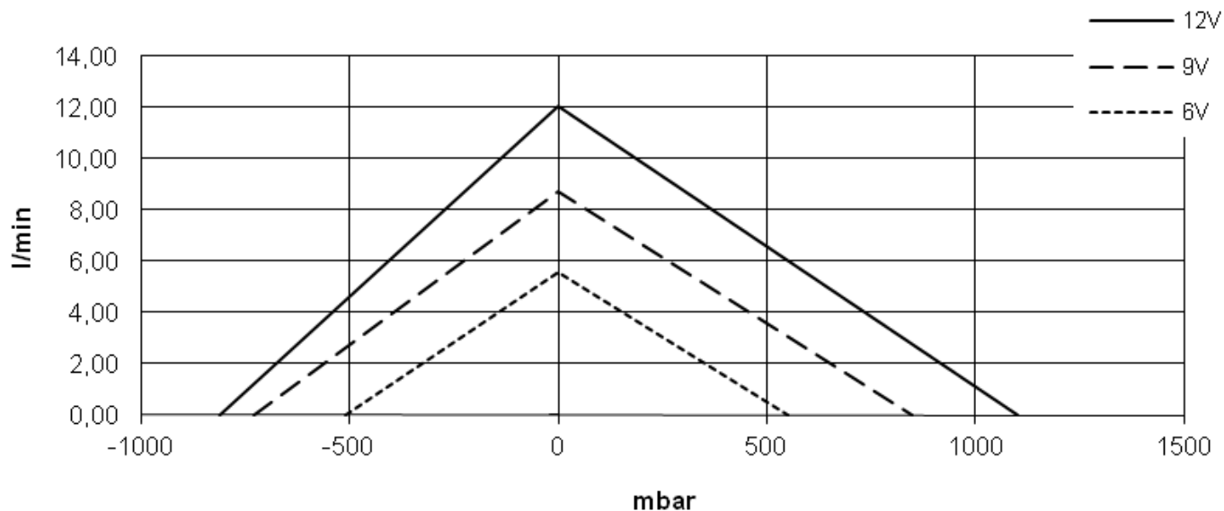
Type/Model: DC12/90L
